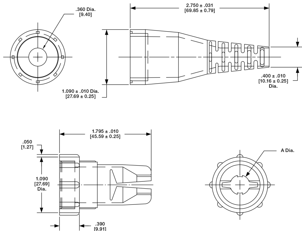
Cable Grip
