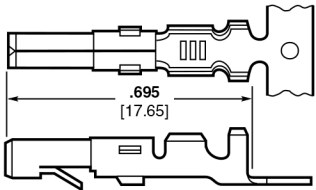
Socket
