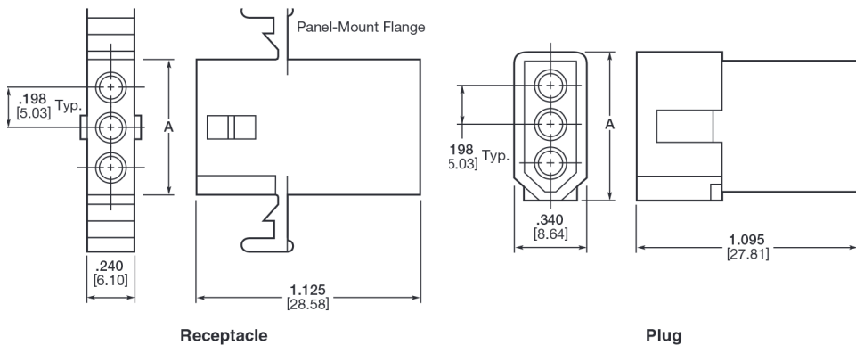
Receptacle
