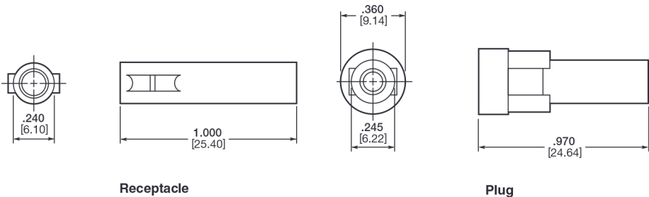
Receptacle
