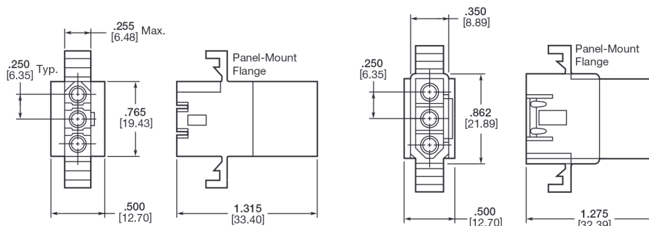
Receptacle
