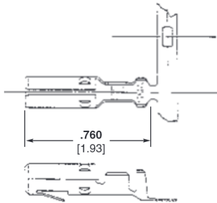
Socket
