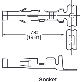
Socket
