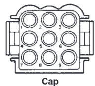
Cap
